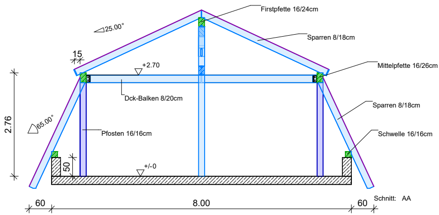
Schnitt A-A
