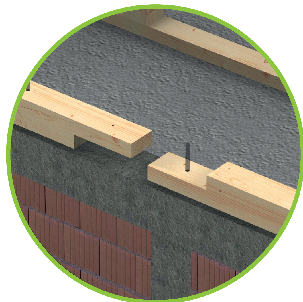
POŁĄCZENIE MURŁAT NA ZAKŁADKĘ
