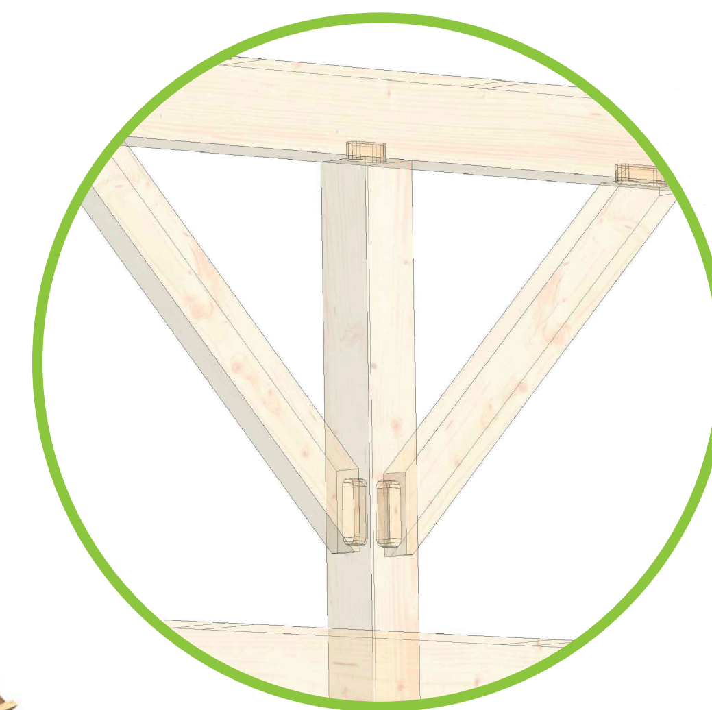
ZASTOSOWANIE CZOPÓW W POŁĄCZENIU ZASTRZAŁÓW ZE SŁUPEM ORAZ PŁATWIĄ
