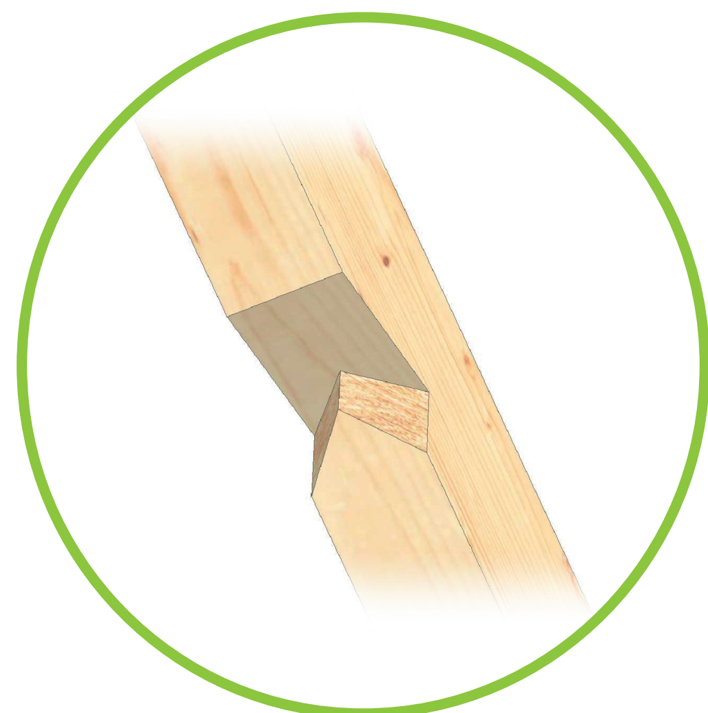
DETAL ZACIOS KROKWI KOSZOWEJ POD PŁATEW
