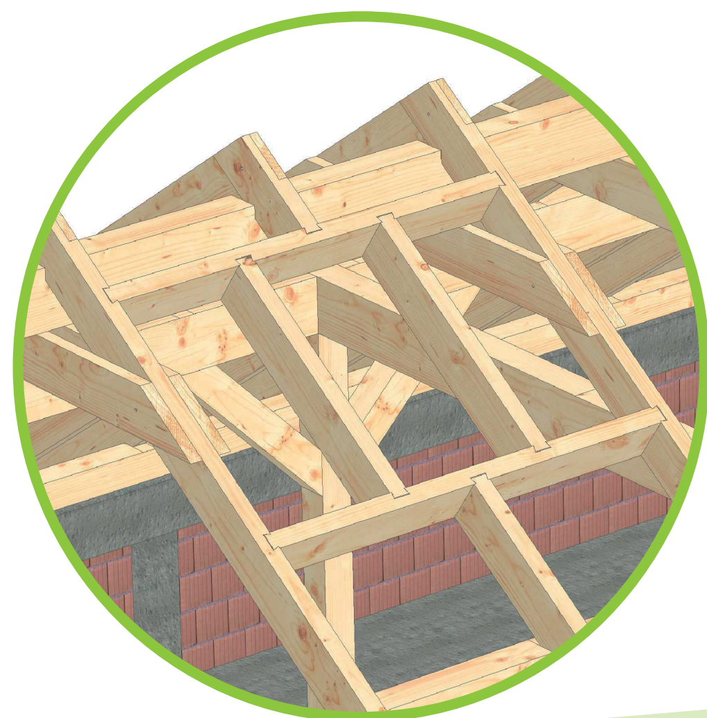
WYMIAN KOMINA Z ZASTOSOWANIEM POŁĄCZEŃ NA „JASKÓŁCZY OGON”
