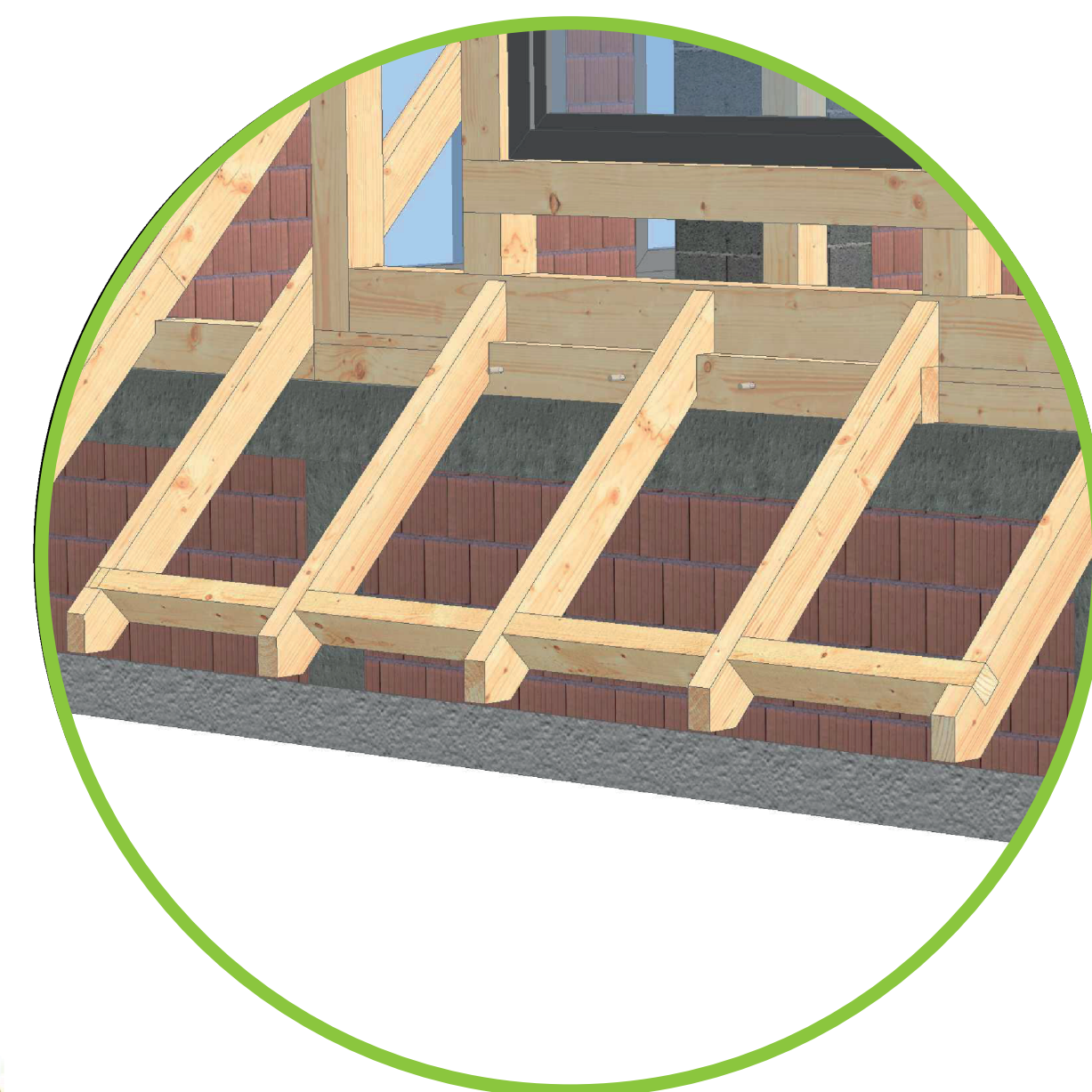
DETAL MOCOWANIE KROKWI KRÓTKICH POD LUKARNĄ
