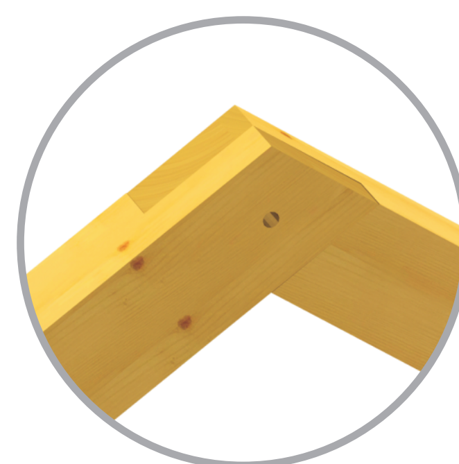
Połączenie na zakładkę prostą
