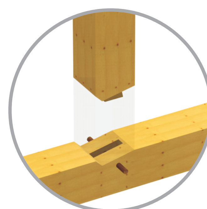
Złącze kątowe na wręb czołowy z czopem i kołkiem
