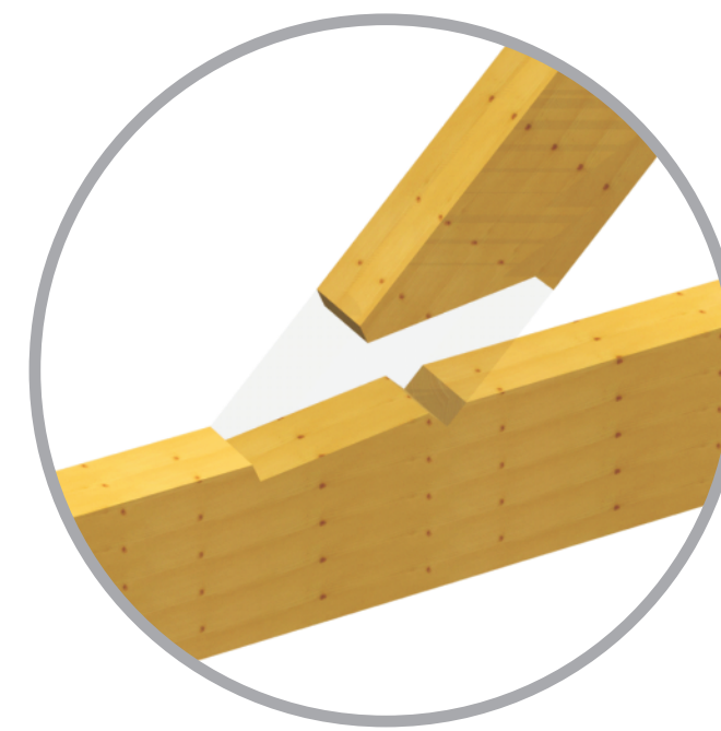
Złącze kątowe na wręb czołowy podwójny
