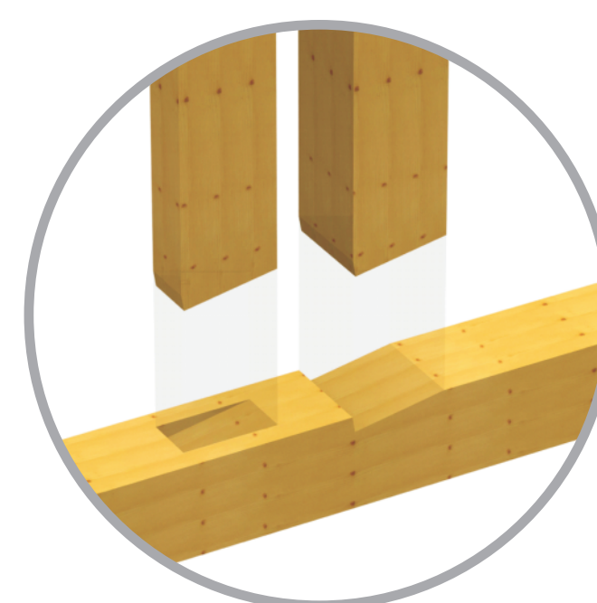
Złącza kątowe na wręb czołowy przedni
