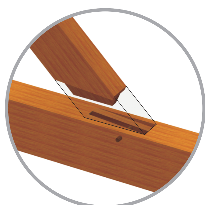
Złącze kątowe na wręb
