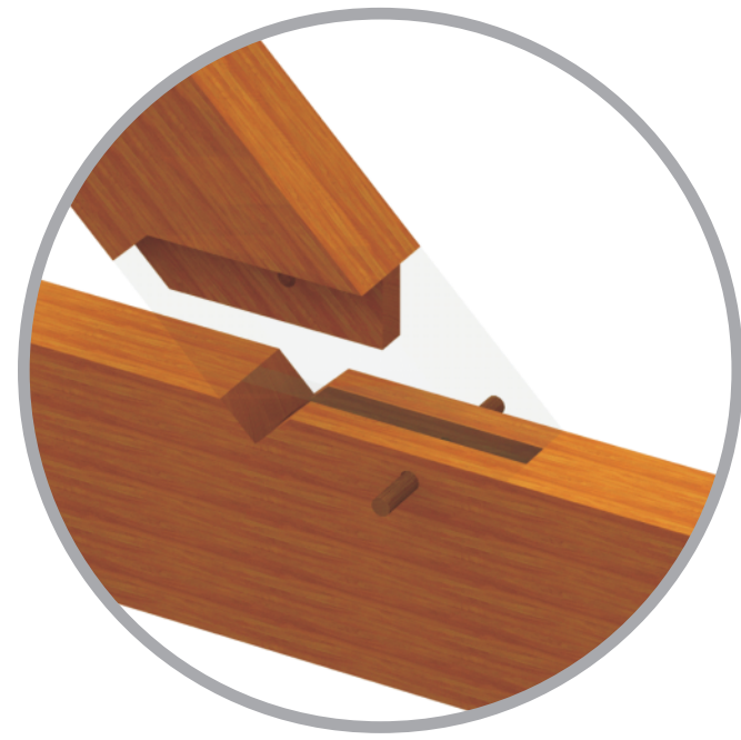
Złącze kątowe na wcięcie z czopem i kołkiem
