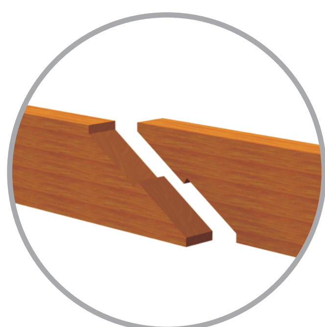
Złącze wzdluzne na zamek ukośny
