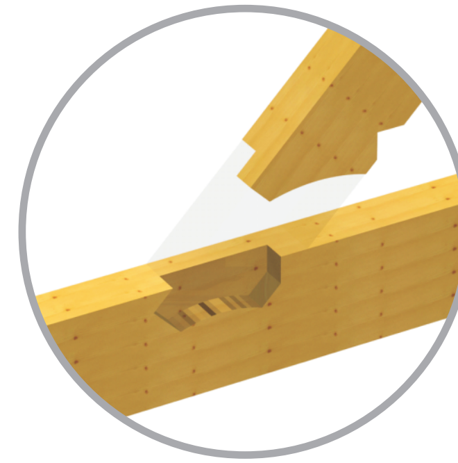
Złącze na zakładkę jaskółczego ogona
