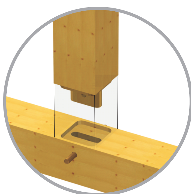
Połączenie na podwójny czop
